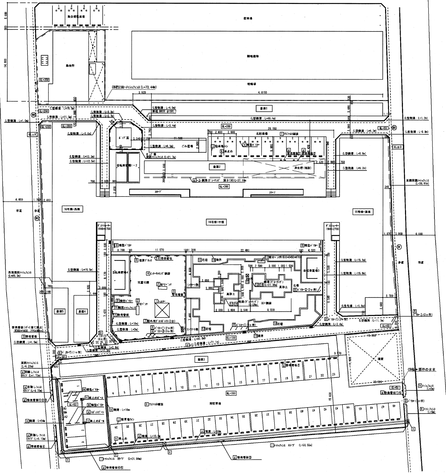
東大阪市荒本住宅16号棟 配置図 1/200
